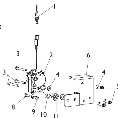
POTENZIOMETRO SUPERIORE UPPER POTENTIOMETER
